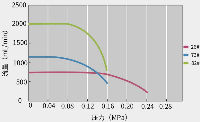
YZ35-II泵头压力曲线图 (100rpm)
